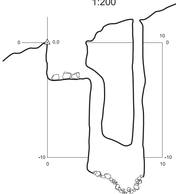
Przekrój (Aufriss) S - N 1:200
